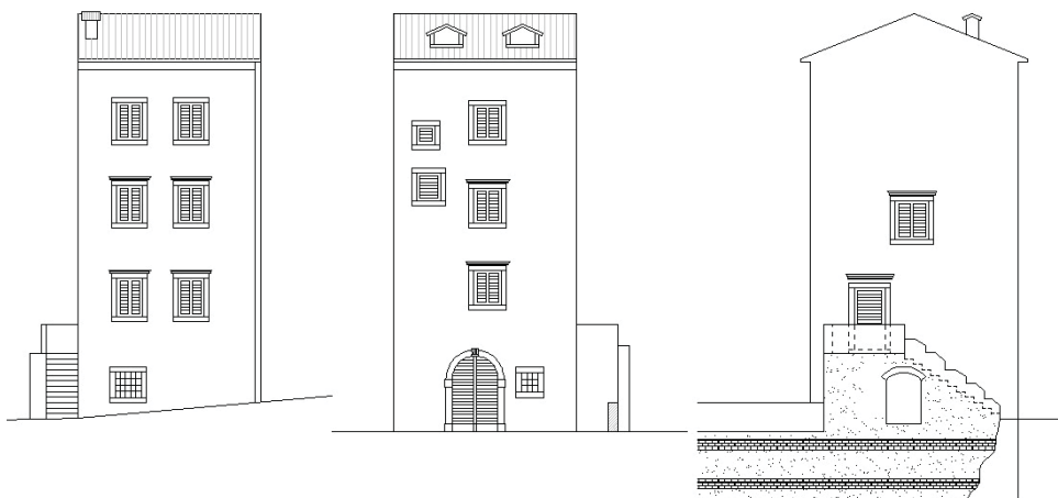
Sjeverno, južno i istočno pročelje – novo stanje
