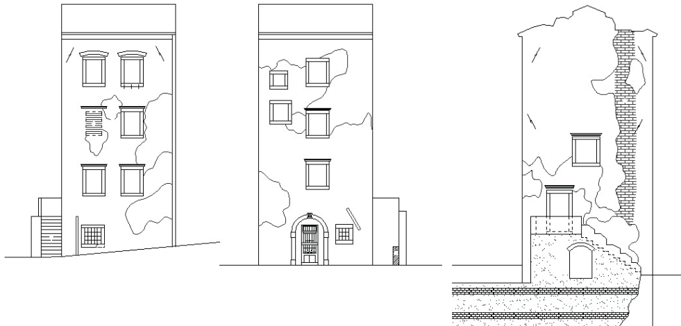
Sjeverno, južno i istočno pročelje – postojeće stanje
