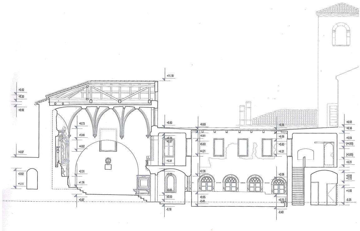
uzdžni presjek
