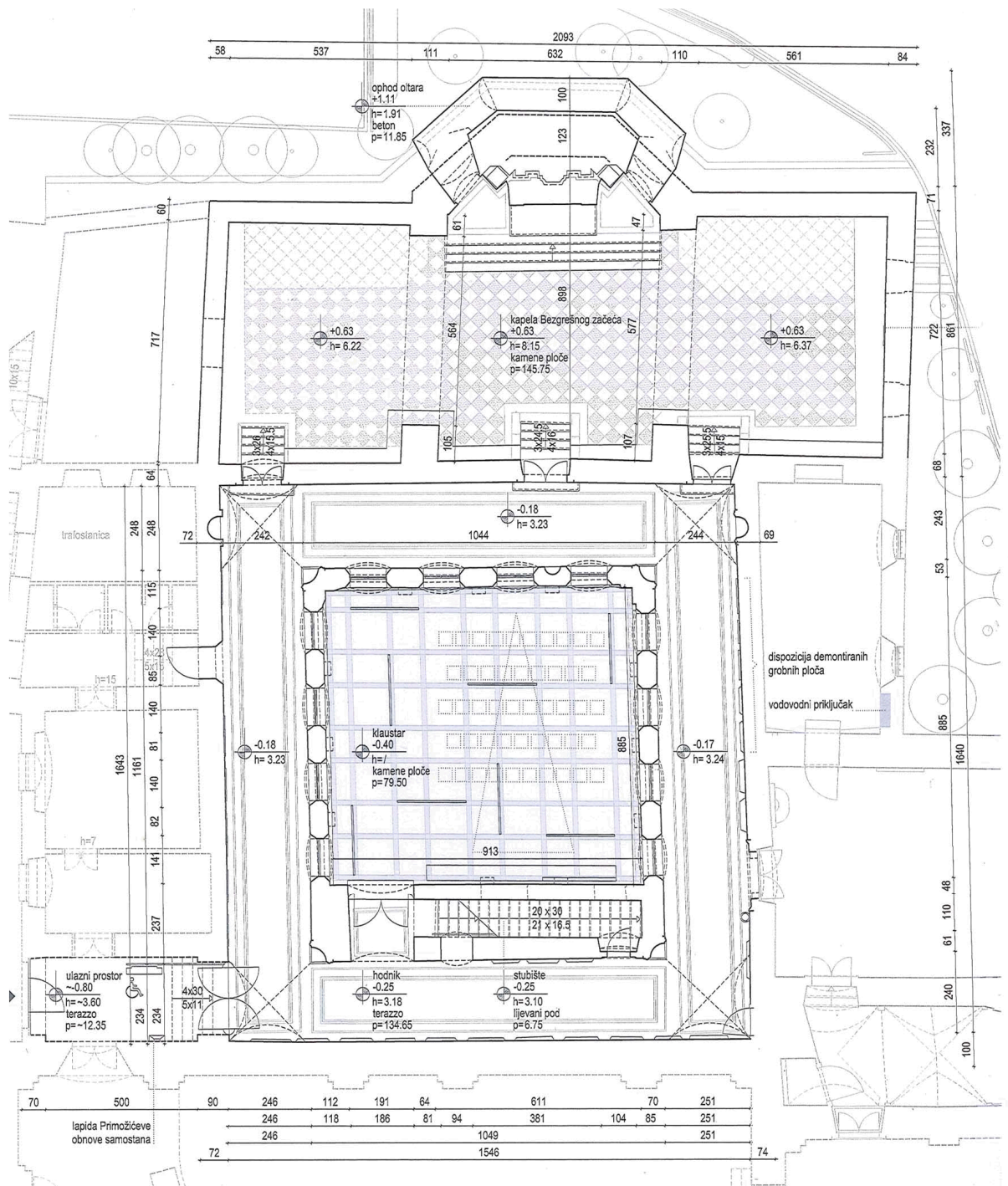
tlocrt prizemlja
