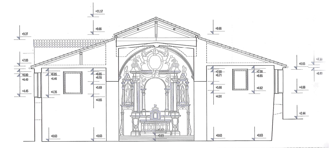
poprečni presjek
