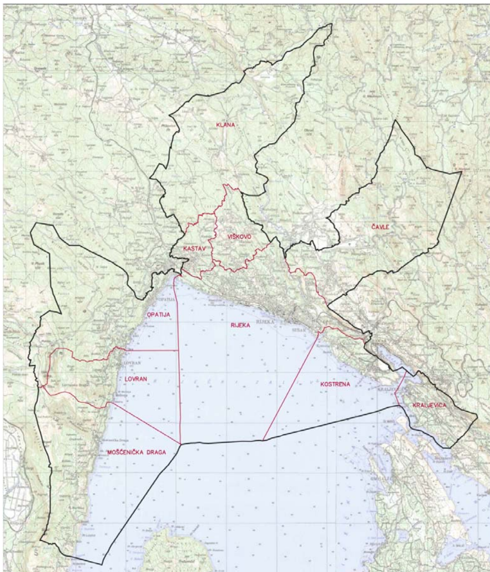
Slika 1. Konačni teritorijalni obuhvat UA Rijeka
