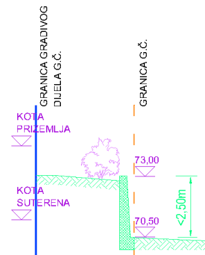
PRESJEK AA POTPORNİ ZİD M 1:200
