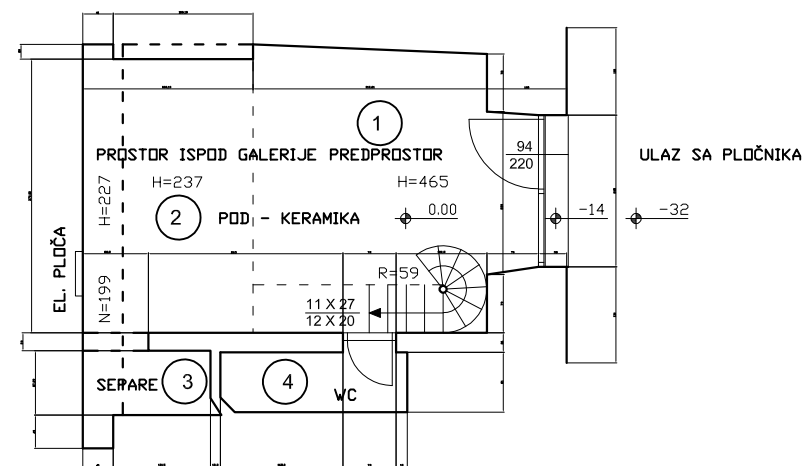
PRIZEMLJE
