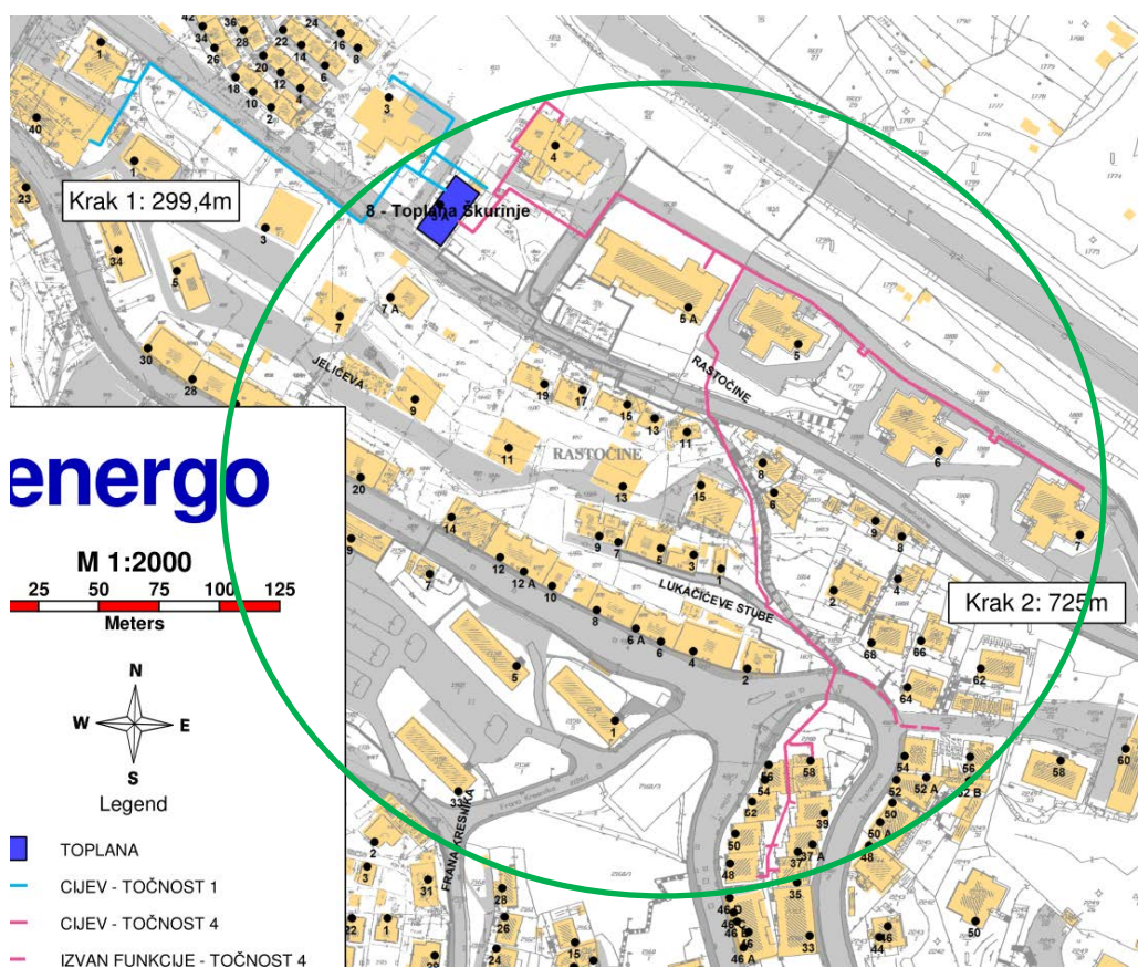
Slika 8: Izvedeni radovi – sustav Skurinjje
