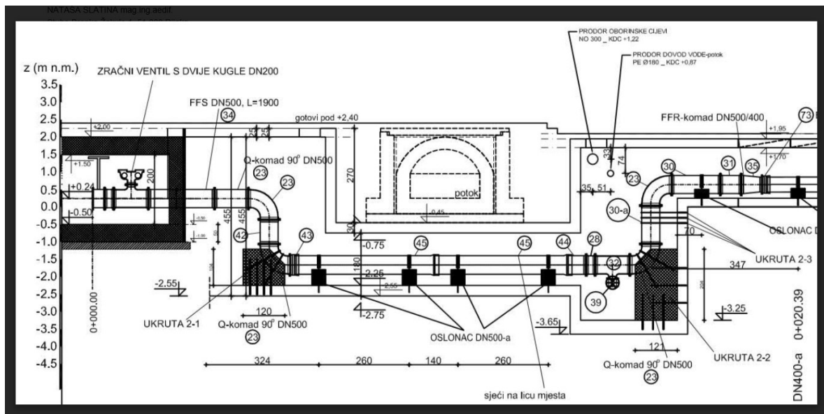
slika 1 - prikaz sifonskog prolaza iz izvedbenog projekta
