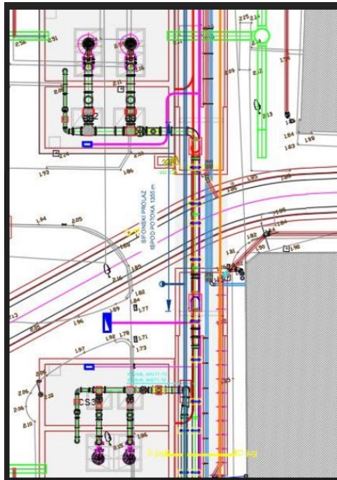
slika 2 - sintezne situacije instalacija
