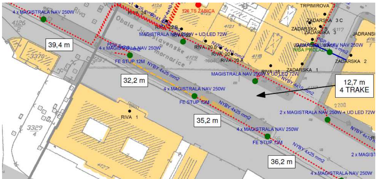
Slika 1: Postojeće stanje javne rasvjete izvedeno pomoću rasvjetnih tijela 4xMAGISTRALA 250W
