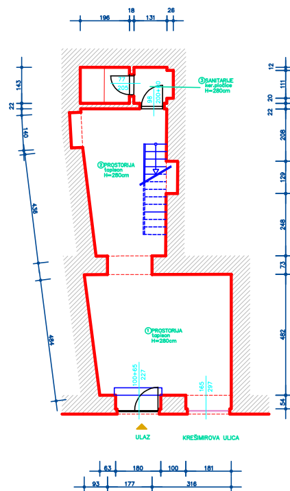
TLOCRT PRIZEMLJA
