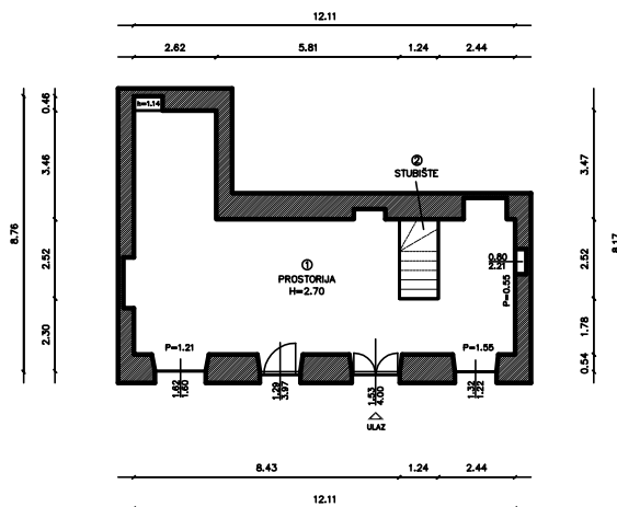
PRIZEMLJE
