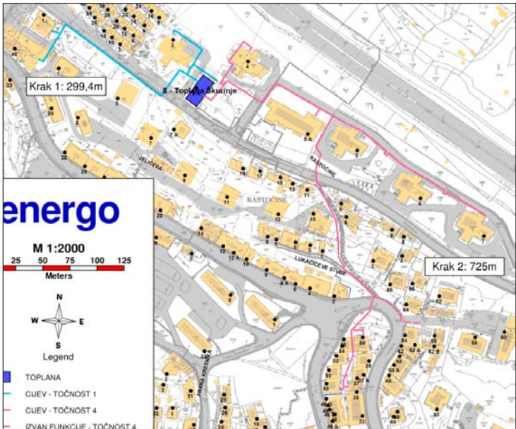
Slika 3. Izvedeni radovi – sustav Škurinje
