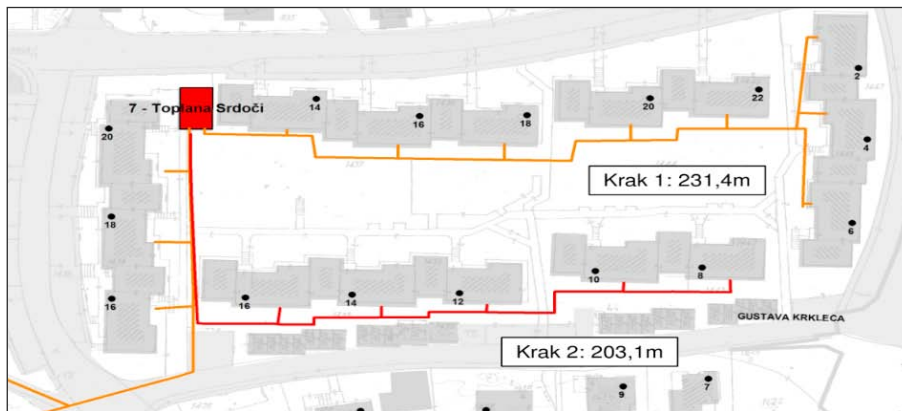
Slika 1. Izvedeni radovi – sustav Srdoči
