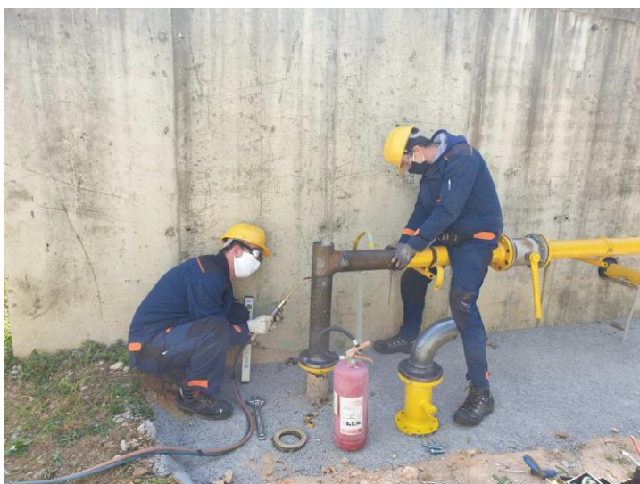
Slika 11: Izrada plinske instalacije za punionicu na lokaciji Milutina Barača
