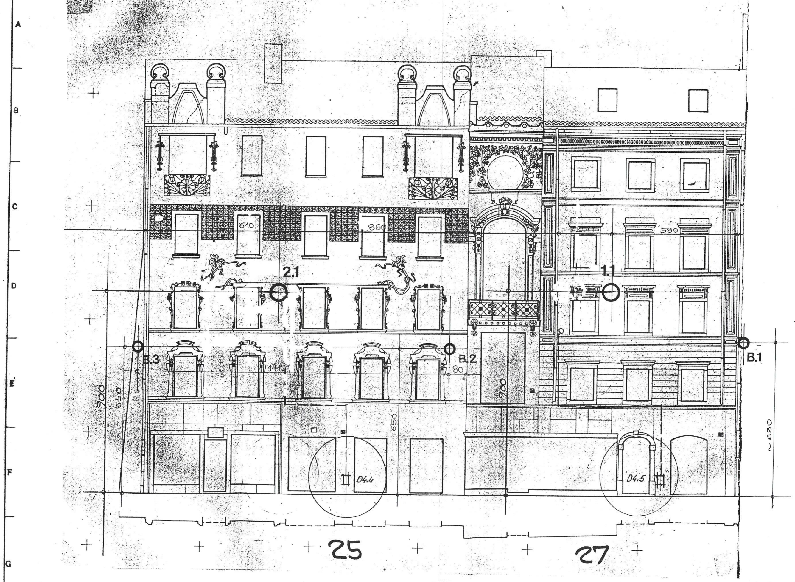
7. MJESTA SIDRIŠTA UŽADI 1:100 LIJEVA STRANA KORZA - br. 25 i 27
