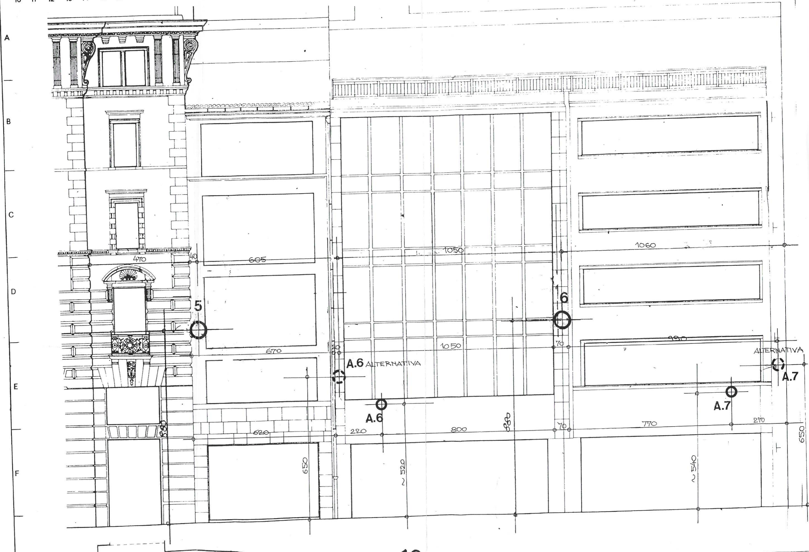
14. MJESTA SIDRIŠTA UŽADI 1:100 DESNA STRANA KORZA - br. 12 i 14
