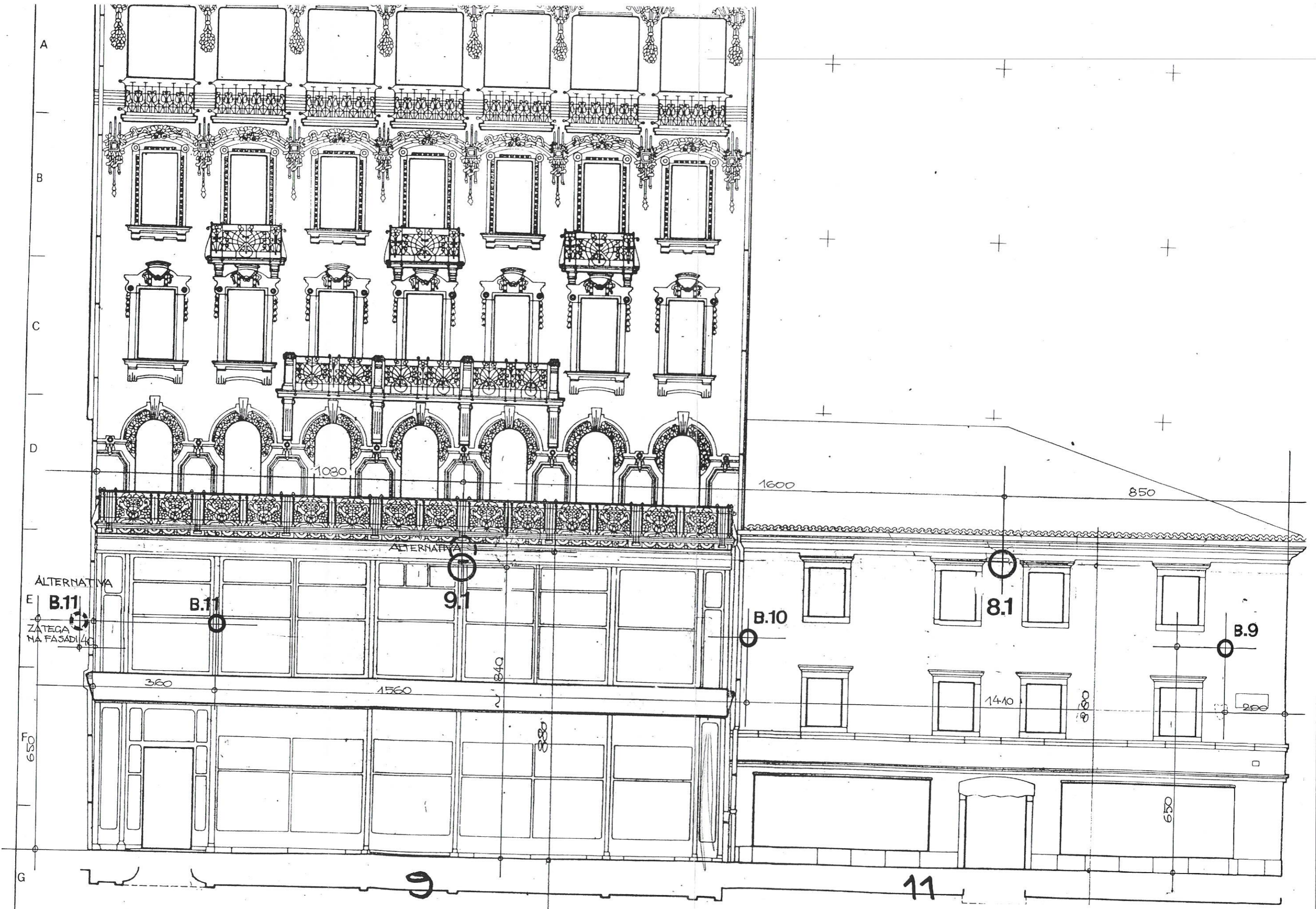
4. MJESTA SIDRIŠTA UŽADI 1:100 LIJEVA STRANA KORZA - br. 9 i 11
