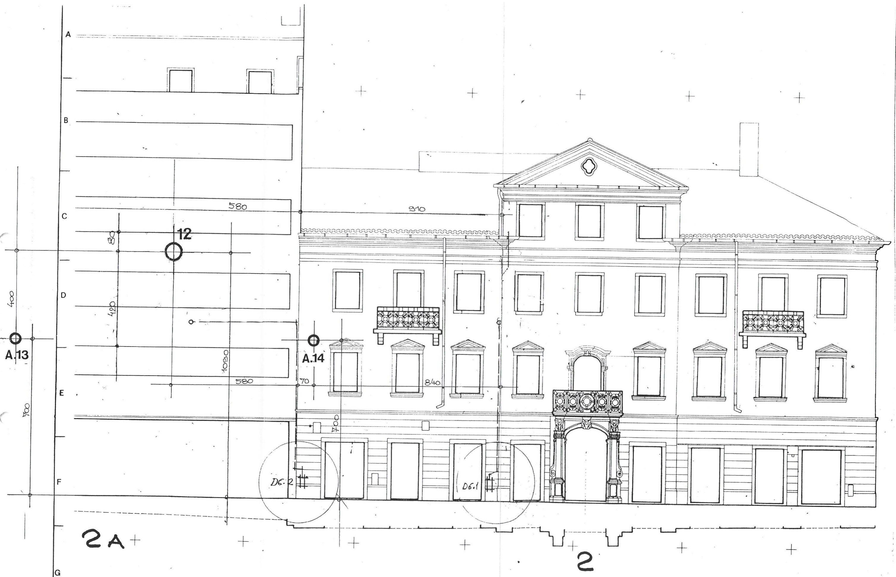
9. MJESTA SIDRIŠTA UŽADI 1:100 DESNA STRANA KORZA - br. 2 i 2a
