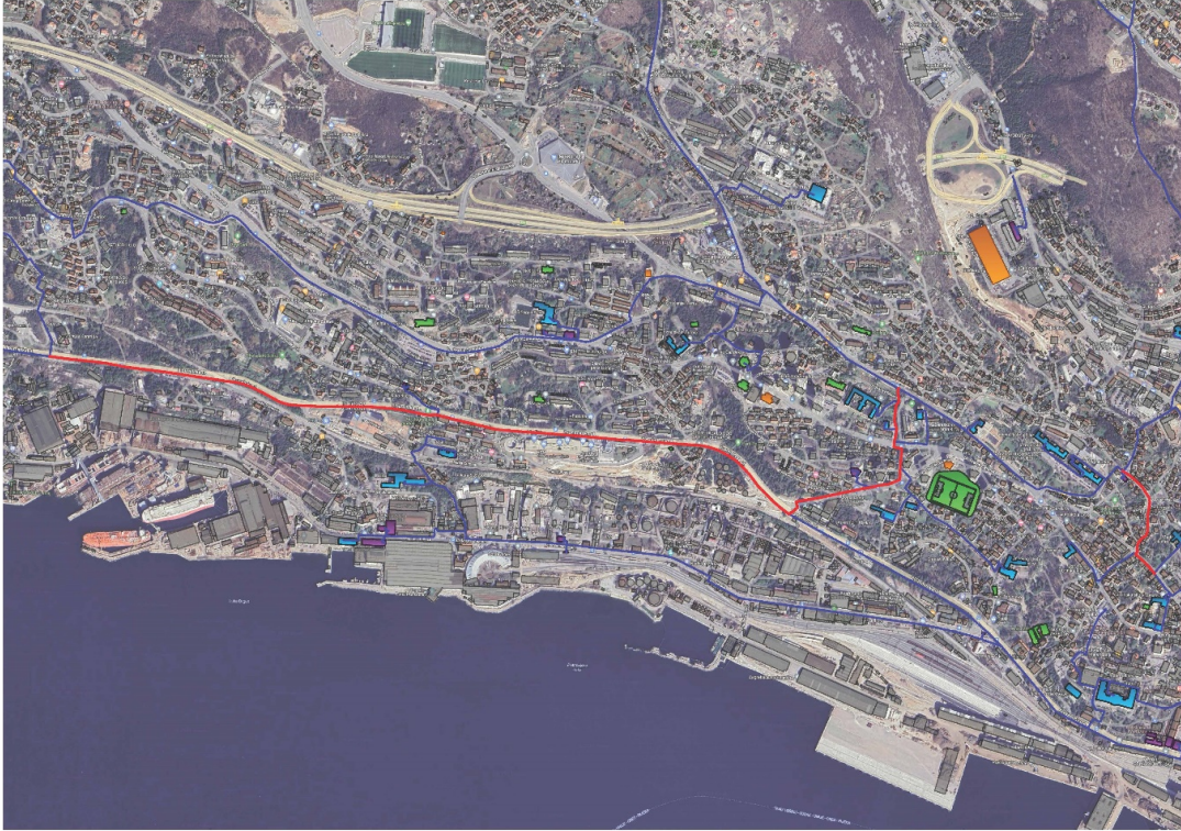
Uris planirane trase svjetlovodnog kabela – smjer „Kantrida - Zamet“ (crveno)
