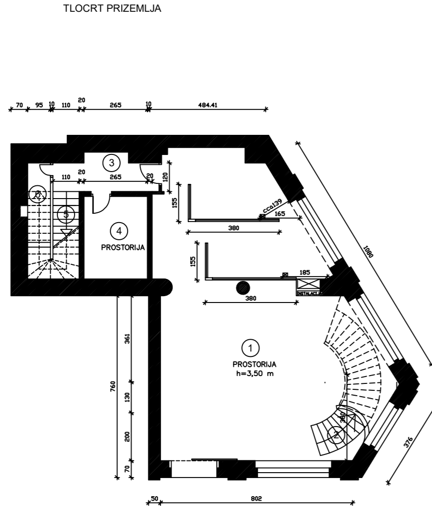
TLOCRT PRIZEMLJA
