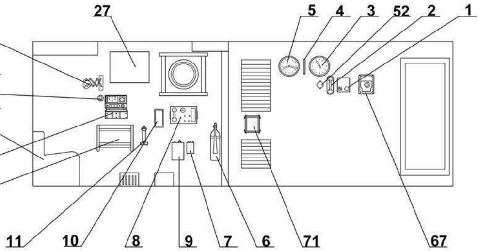
POGLED NA KRMENU STIJENU
