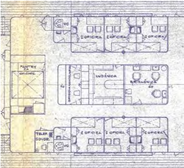
Smještaj i arhivski nacrt prostorije 41
