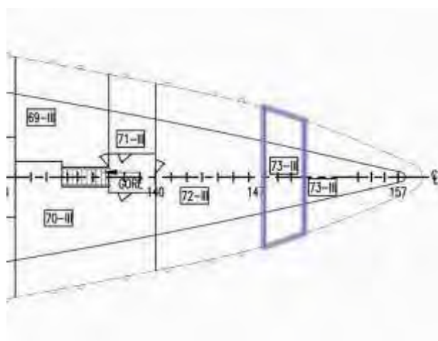
Smještaj i arhivski nacrt prostorije 132
