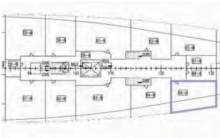
Smještaj i arhivski nacrt prostorije
