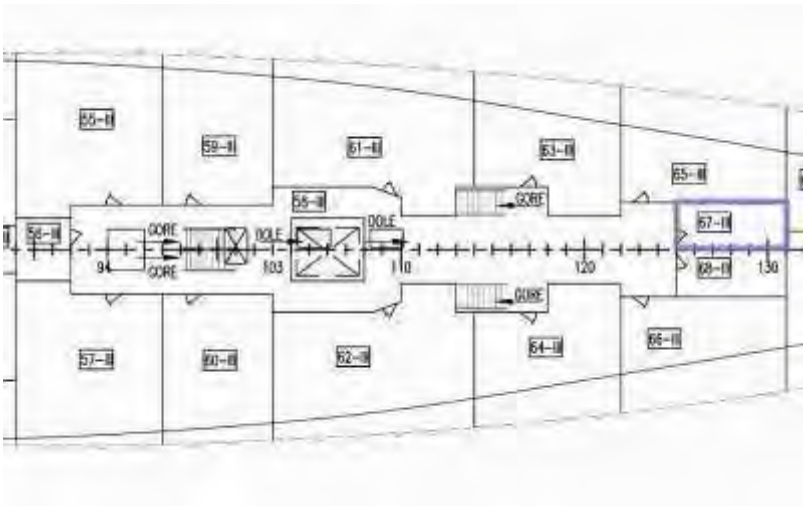
Smještaj i arhivski nacrt prostorije
