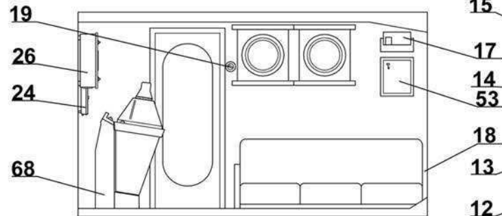
POGLED NA DESNU BOČNU STIJENU
