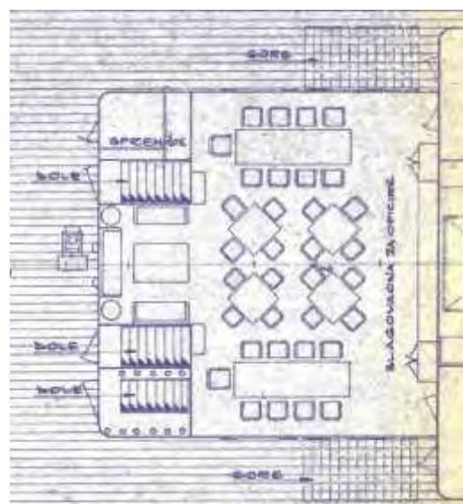
Smještaj i arhivski nacrt prostorije 39
