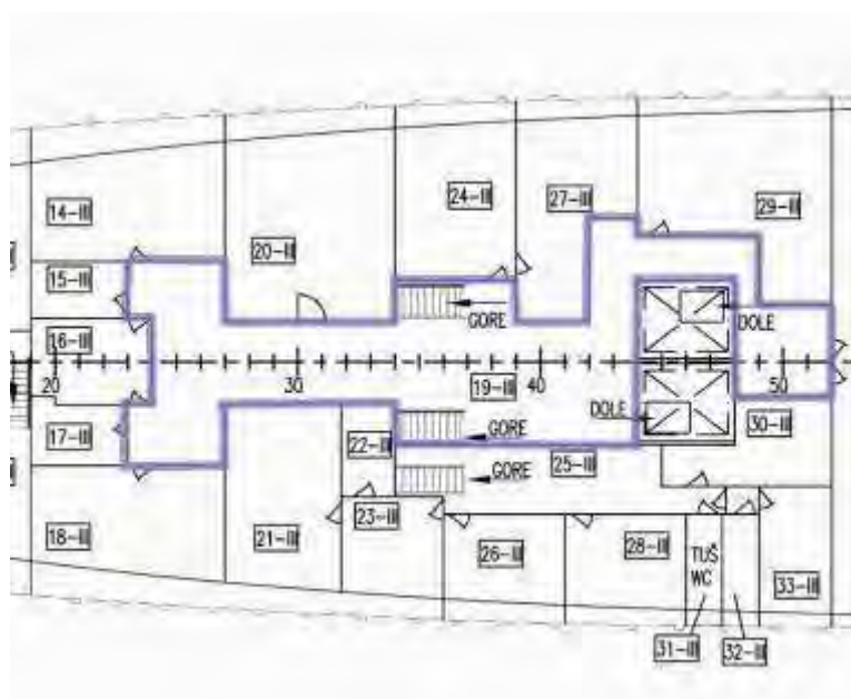
Smještaj i arhivski nacrt prostorije 95
