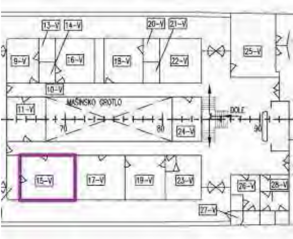
Smještaj i arhivski nacrt prostorije 31
