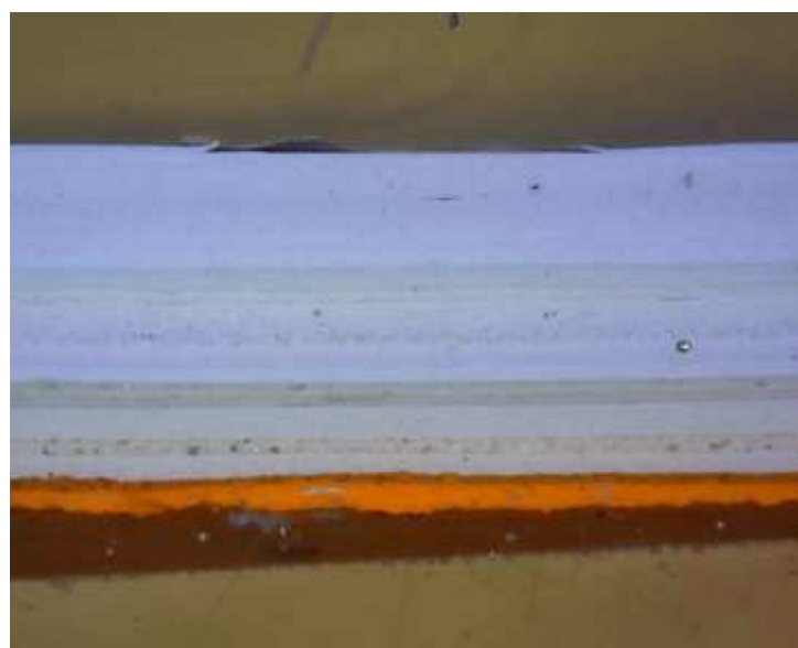
Slika 63 a, b, Izrada mikropresjeka uzorka bojanog sloja, izvor: eLABORO d.o.o.
