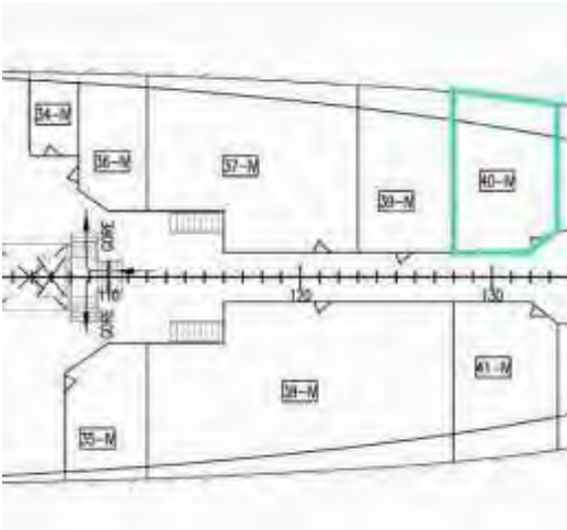
Smještaj i arhivski nacrt prostorije 76
