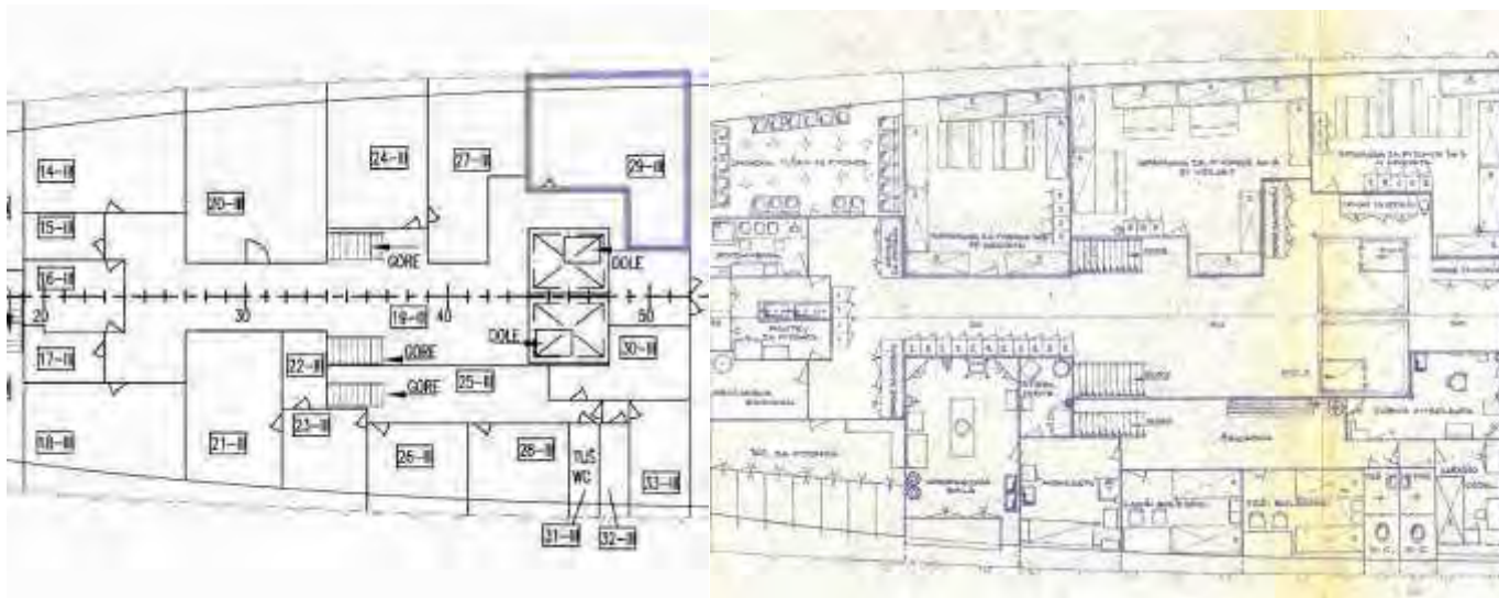
Smještaj i arhivski nacrt prostorije 103
