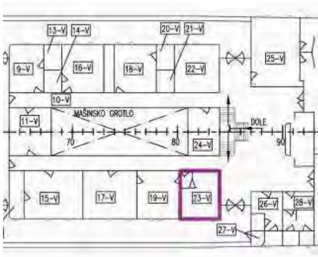
Smještaj i arhivski nacrt prostorije V-23
