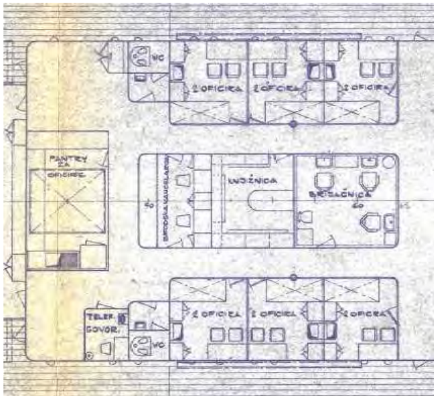
Smještaj i arhivski nacrt prostorije 48
