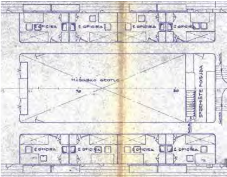
Smještaj i arhivski nacrt prostorije 55
