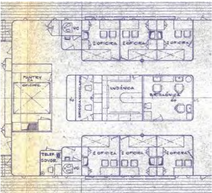
Smještaj i arhivski nacrt prostorije 51
