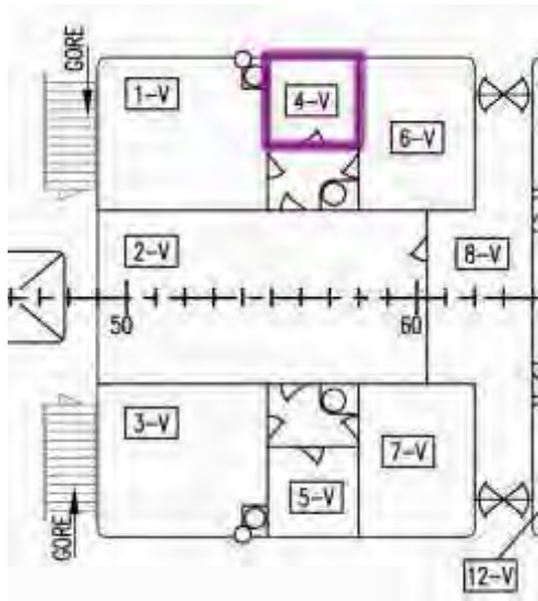
Smještaj i arhivski nacrt prostorije 23
