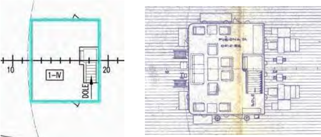
Smještaj i arhivski nacrt prostorije 37
