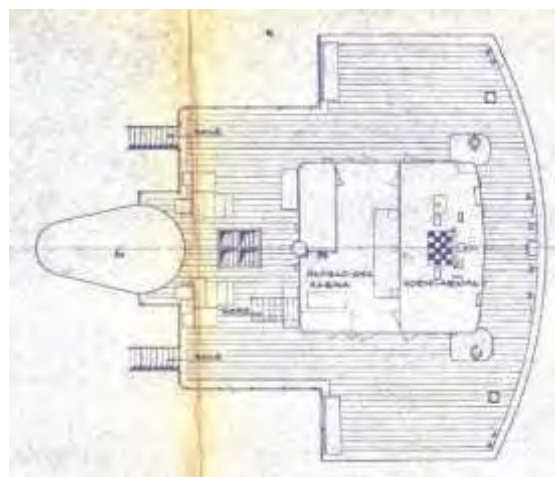
Smještaj i arhivski nacrt prostorije 5
