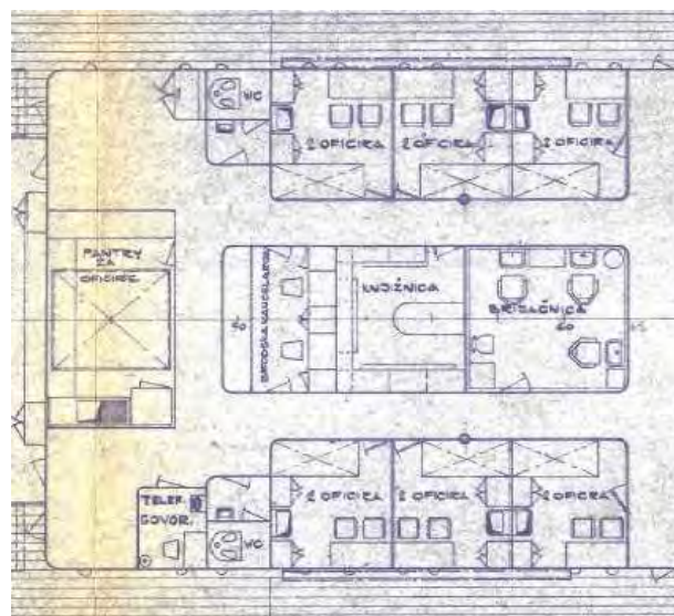
Smještaj i arhivski nacrt prostorije 47
