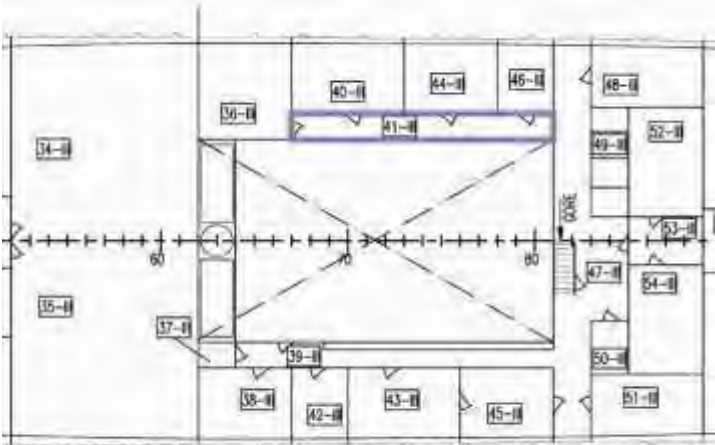
Smještaj i arhivski nacrt prostorije 114
