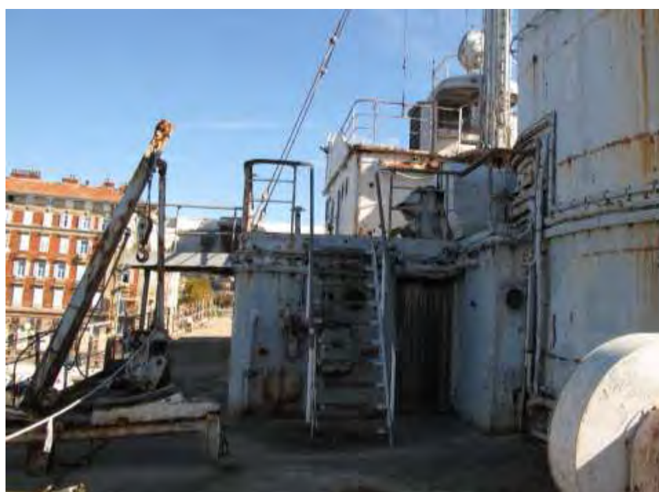
Slika 40, Bočni dio otvorenog dijela palube čamaca s pogledom na nadgrađe zapovjednog mosta, izvor: eLABORO d.o.o.
