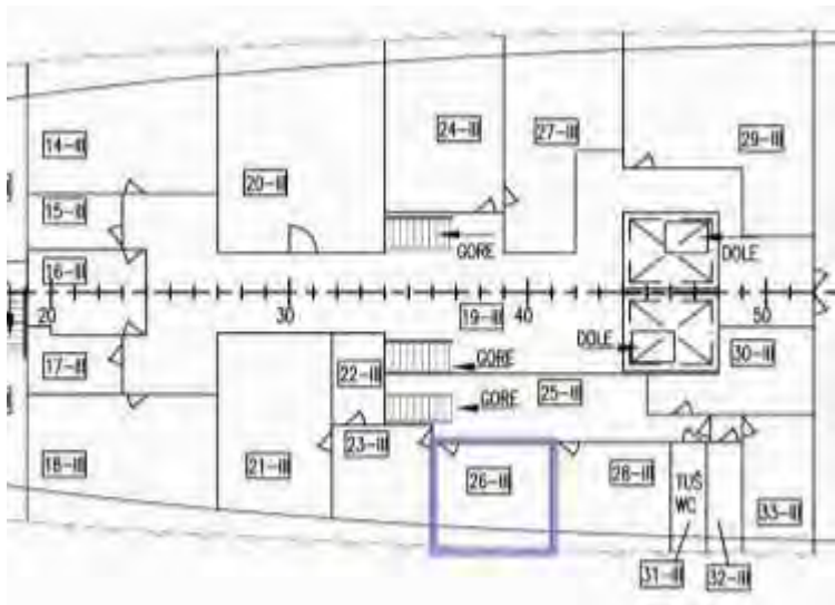
Smještaj i arhivski nacrt prostorije 100
