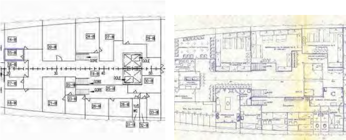
Smještaj i arhivski nacrt prostorije III-12
