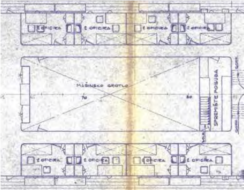
Smještaj i arhivski nacrt prostorije 56
