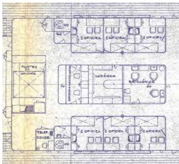
Smještaj i arhivski nacrt prostorije 46
