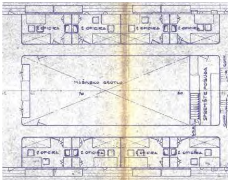
Smještaj i arhivski nacrt prostorije 57
