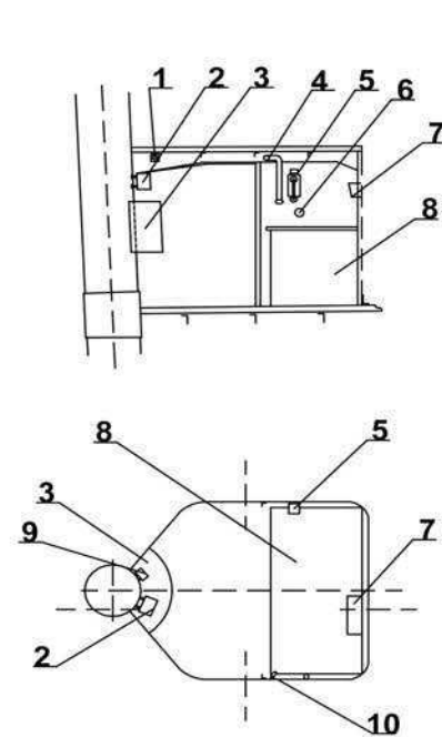
POGLED NA LIJEVU BOČNU STRANU
