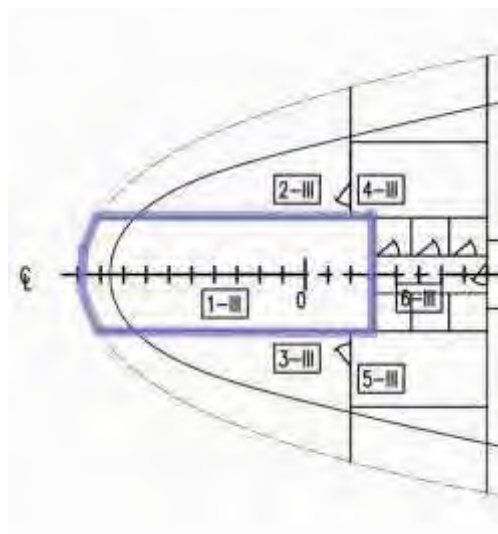
Smještaj i arhivski nacrt prostorije III-1, 2, 3
