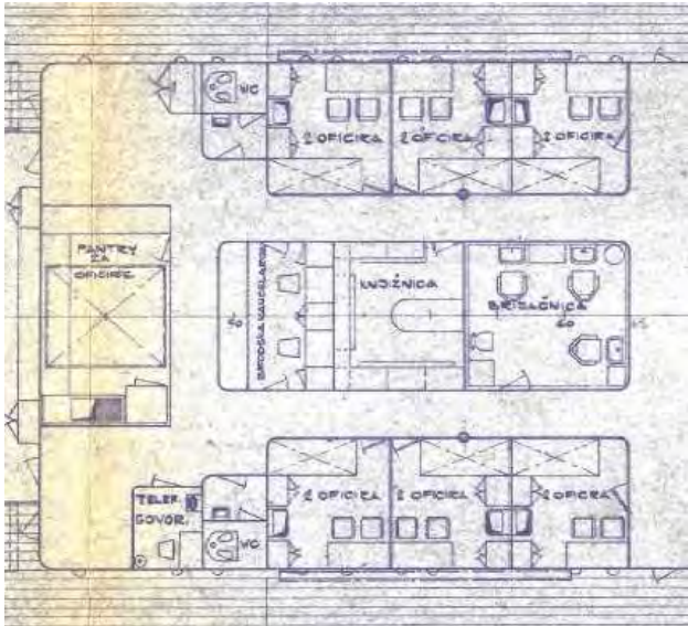
Smještaj i arhivski nacrt prostorije 43
