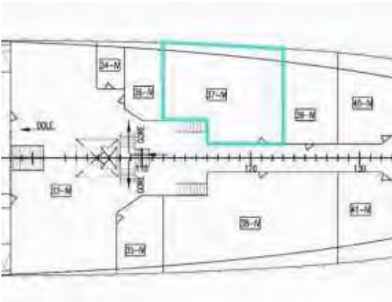
Smještaj i arhivski nacrt prostorije 73
