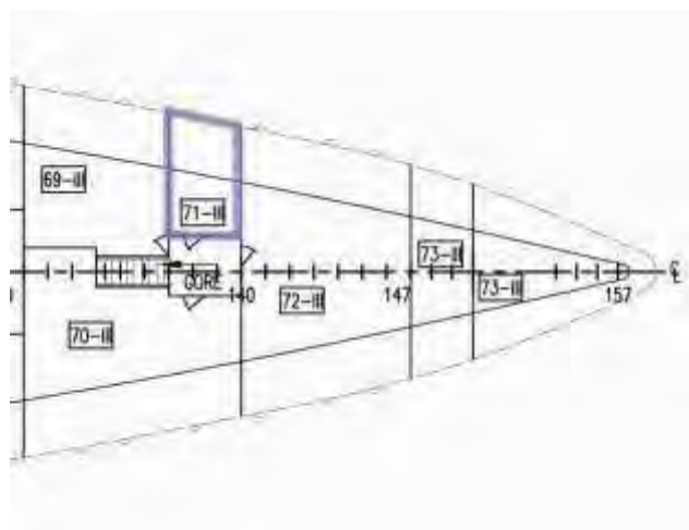
Smještaj i arhivski nacrt prostorije 130
