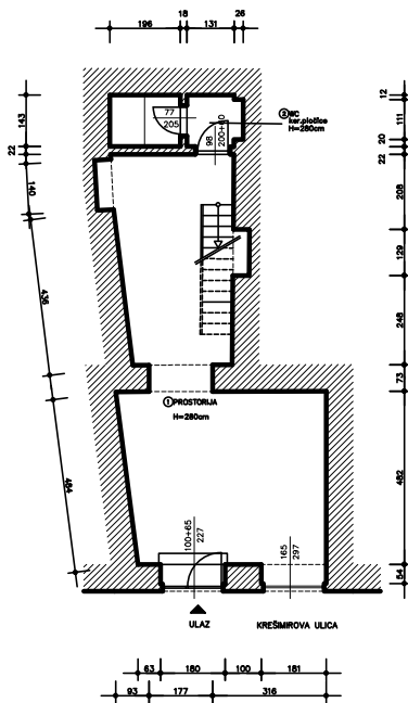
TLOCRT PRIZEMLJA
