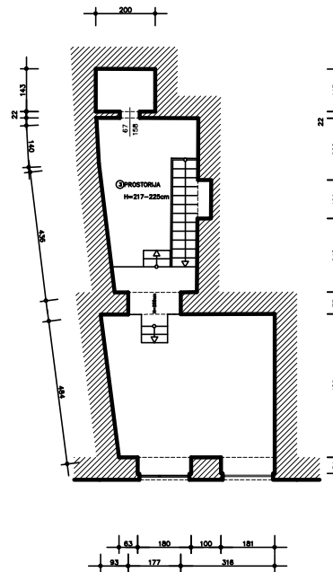
TLOCRT GALERIJE
