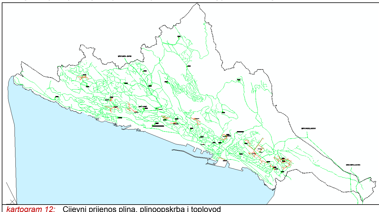
kartogram 12: Cijevni prijenos plina, plinoopskrba i toplovod
